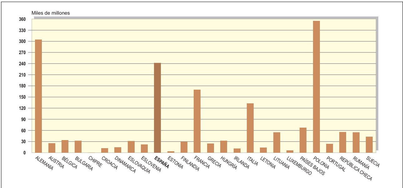
19.3. TRANSPORTE DE MERCANCÍAS POR CARRETERA POR PAÍSES. 2020. (Toneladas/km)
